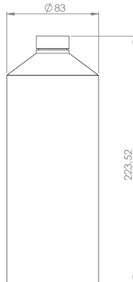
Fig. 4 Vista frontal
