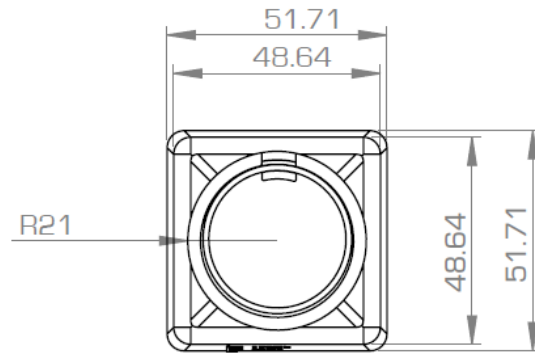
Fig. 2 Vista superior
