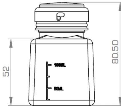
Fig. 1 Vista frontal
