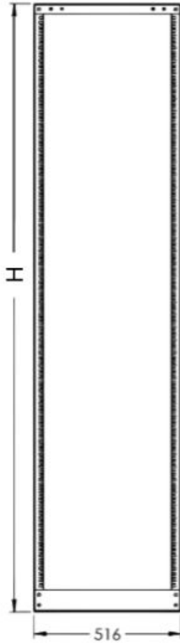
Fig. 2: Vista Frontal
