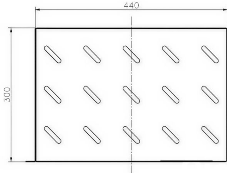
Fig. 2: Vista superior
